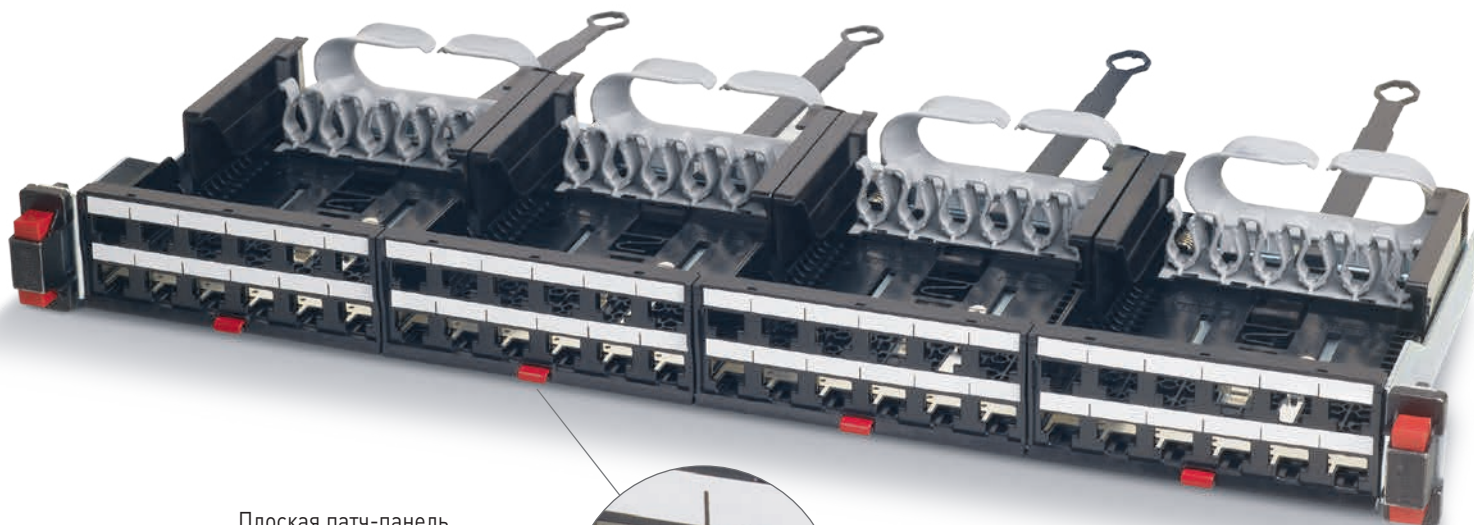
Плоская патч-панель высотой 1U на 48 портов
