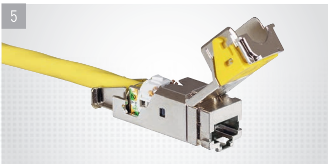
Установить основание в корпус
