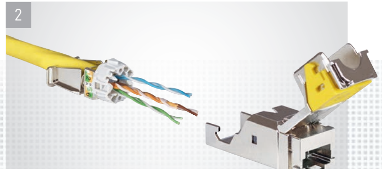
Пропустить пары кабеля сзади через основание коннектора
