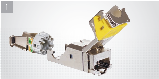
Взять основание коннектора
