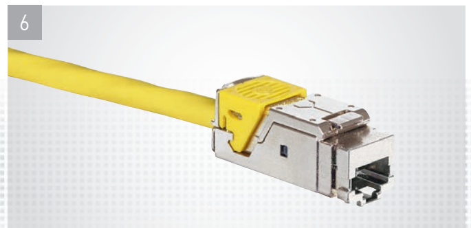
Опустить скобу и защелкнуть коннектор
